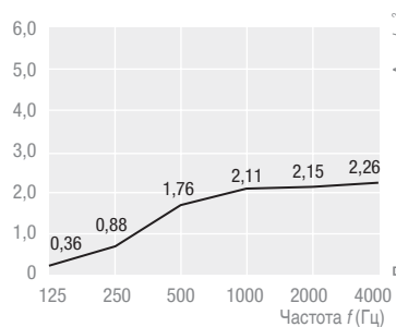
THERMATEX® Sonic element квадратный 1200 x 1200 мм, высота подвеса 150 мм
