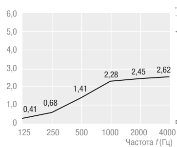
THERMATEX® Sonic element квадратный 1200 x 1200 мм, высота подвеса 300 мм
