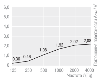
THERMATEX® Sonic element круглый Ø 1200 мм, высота подвеса 300 мм
