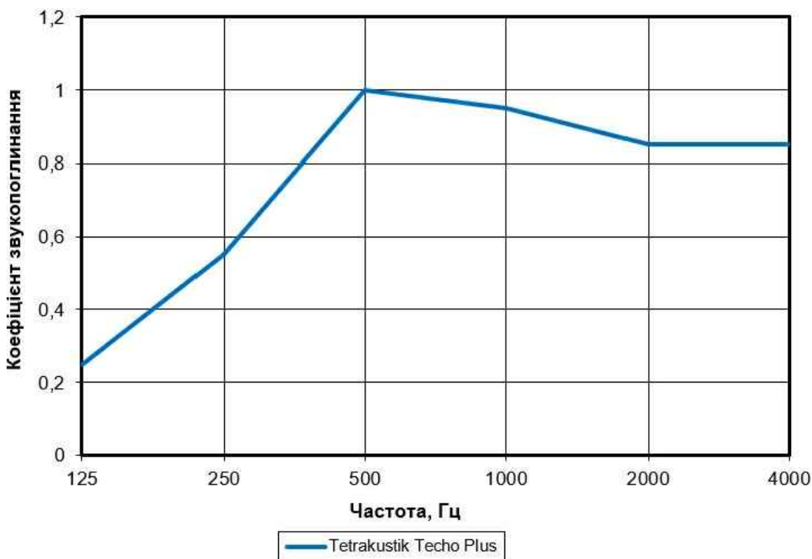
Ревербераційний коефіцієнт звукопоглинання панелями
